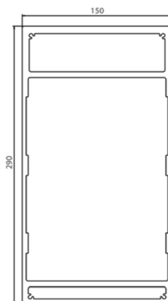
prierez nosníkom
