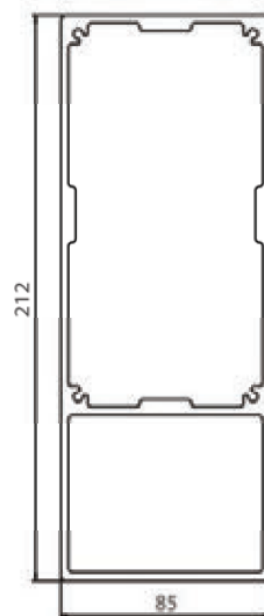
prierez nosníkom
