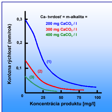
Obr. 2: Protikorózná ochrana
