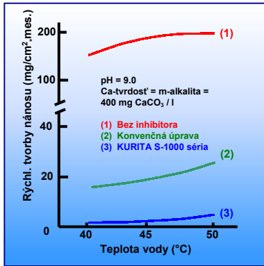
Obr. 1: Stabilizačný účinok
