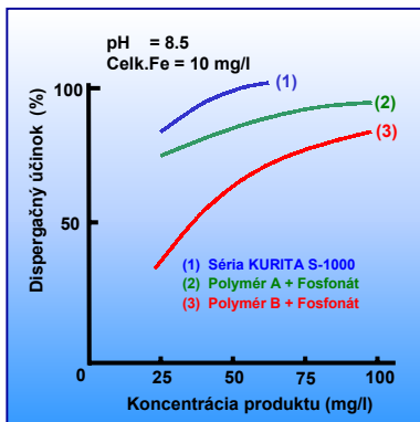
Obr. 3: Dispergácia železa
